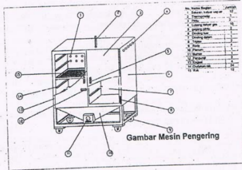
Gambar 1. Sketsa Alat Pengering yang Diperkenalkan
