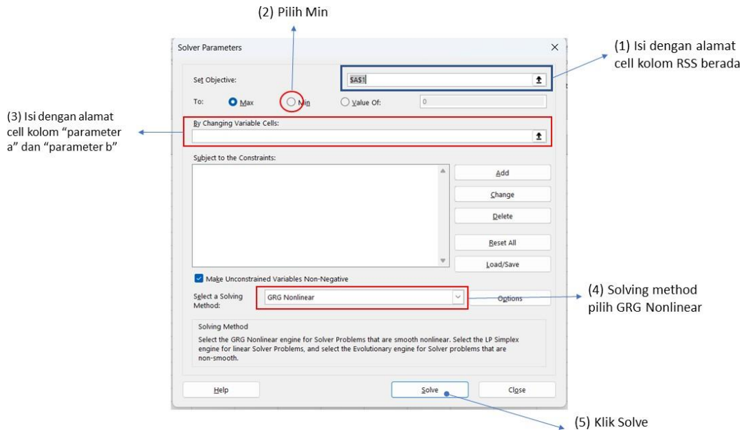
Gambar 1 prosedur penggunaan solver untuk curve fitting
